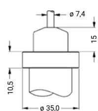
Kabelausgang mit PVC-Kabel 4 (IP 67)
