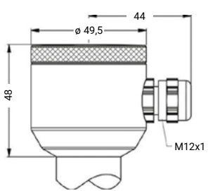
Kompakt-Feldgehäuse (IP 67)
