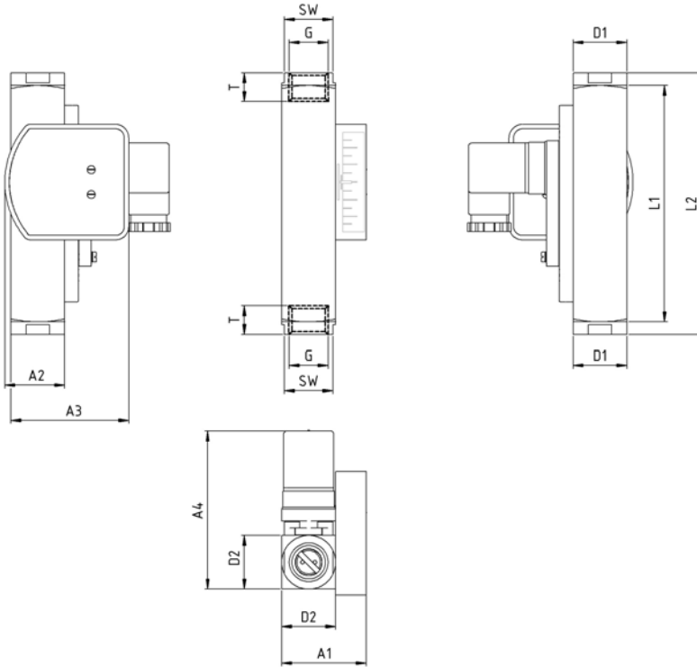
Fig. 70: Type SW-06.X.X.1.08
