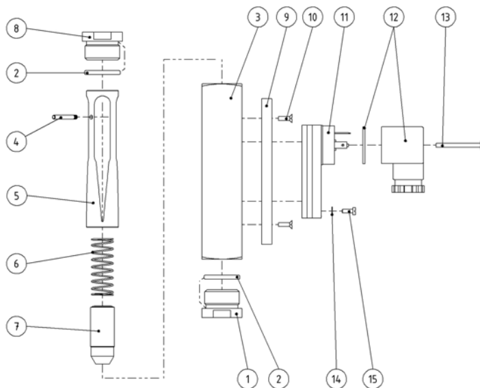
Fig. 61: Type SW-06.X.X.1.08
