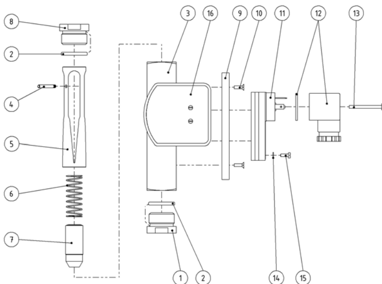
Fig. 73: Type SW-06.X.X.1.08
