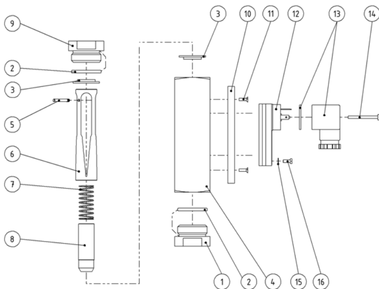
Fig. 62: Type SW-06.X.X.1.10
