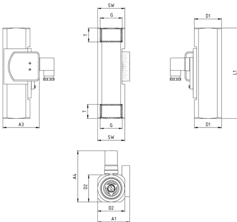
Fig. 72: Type SW-06.X.X.1.13a und SW-06.X.X.1.14
