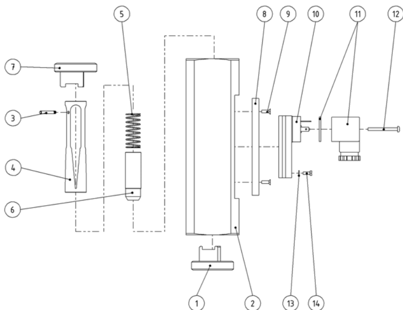
Fig. 75: Type SW-06.X.X.1.13a und SW-06.X.X.1.14
