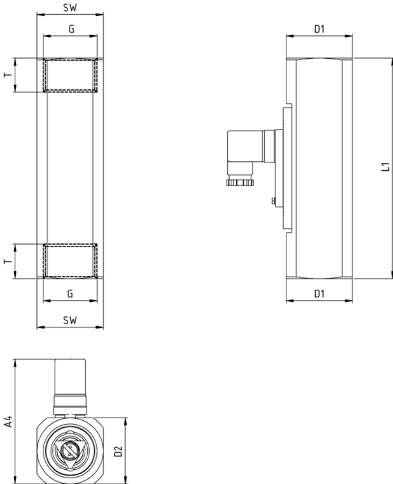
Fig. 60: Type SW-06.X.X.1.13a und SW-06.X.X.1.14
