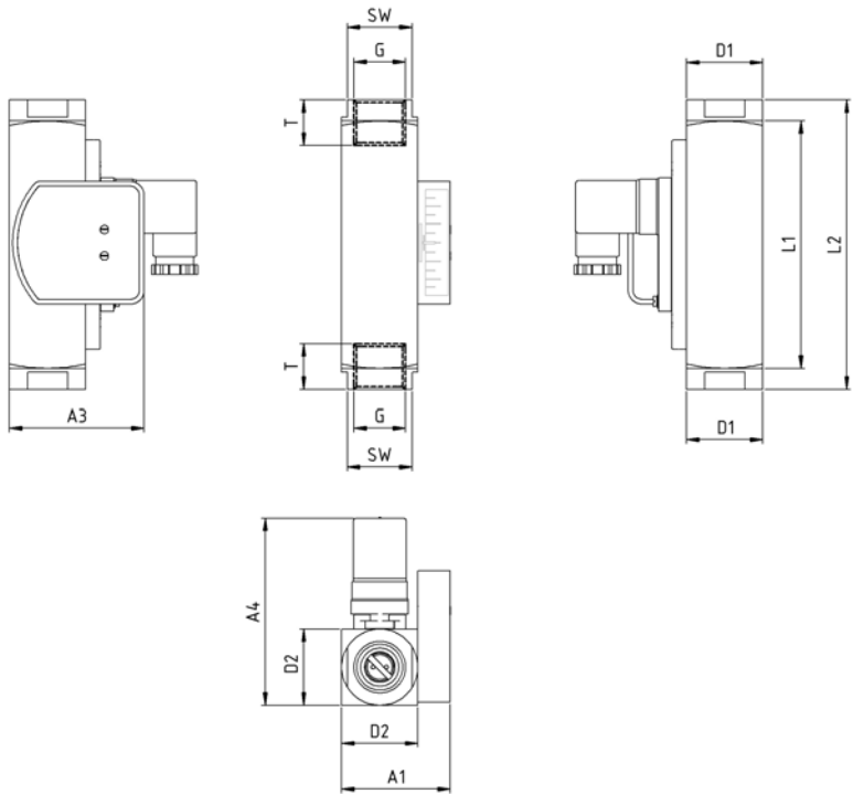
Fig. 71: Type SW-06.X.X.1.10
