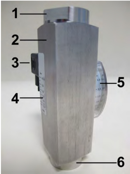
Fig. 2: SW-06 overview
